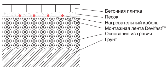
Бетон (кабель в песке)
